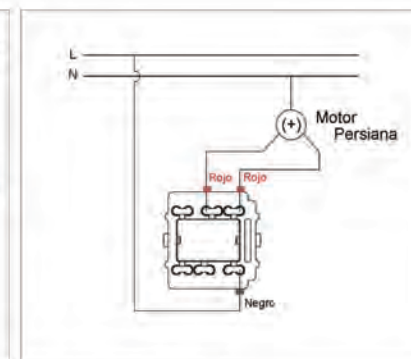
Mecanismos para persianas Electric blinds mechanism
